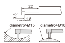
sensor de superfície curva (opcional), código ISR-C002-SUR
