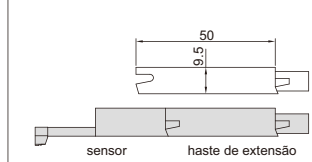
haste de extensão (opcional), código ISR-C002-ER
