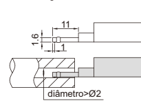
tiny hole probe (opcional), código ISR-C002-SBP
