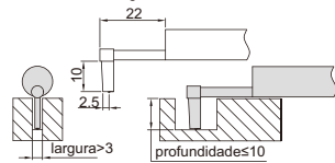
sensor para rebaixo profundo (opcional), código ISR-C002-DGP
